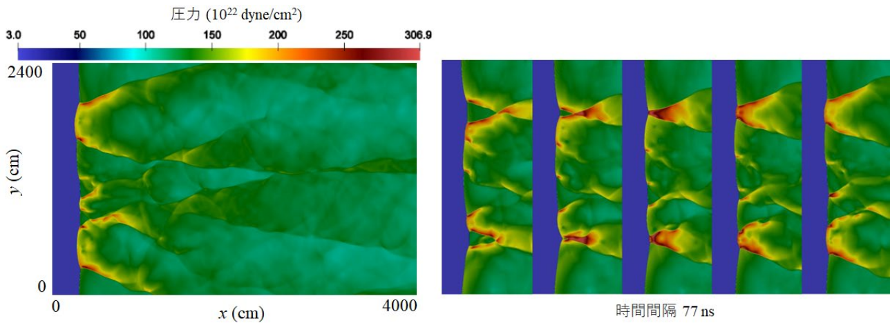
図1 セル構造シミュレーション結果の例。密度 1 \times 10^6 \text{ g/cm}^3 、ヘリウム質量分率 0.6 における圧力分布：(左)計算領域全体の瞬間図 (右)77ns 間隔の連続図
