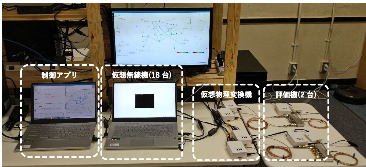
図 3：仮想空間で動作する無線機と物理無線機(評価機)の相互接続
