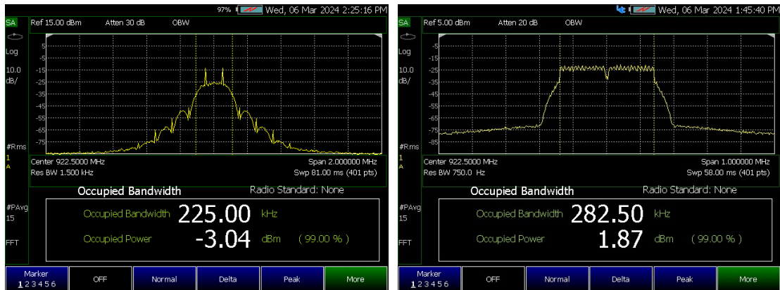
図 2：評価基板の出力波形(左：FSK、右：OFDM) 受信信号をアッテネータで減衰後にスペクトルアナライザで測定
